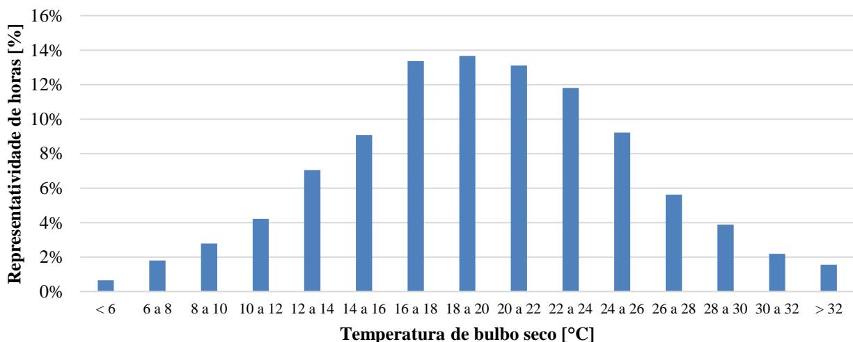
Figura 2. Temperatura de bulbo seco para todas as horas do ano em Rio Pardo.
