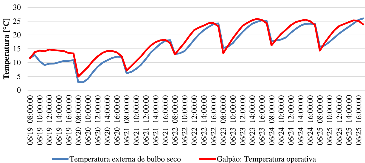
Figura 4. Comportamento da temperatura operativa no Caso 1 para semana típica de inverno de projeto.
