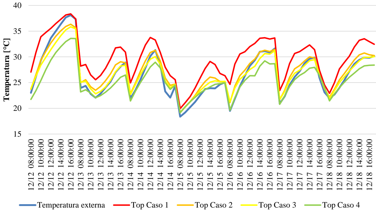
Figura 6. Comparação da temperatura operativa dos casos de envoltória para a semana típica de verão de projeto.
