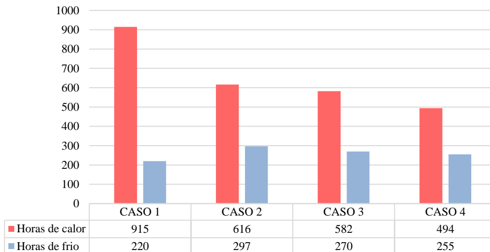
Figura 8. Comparação de horas de desconforto entre os casos de envoltória.
