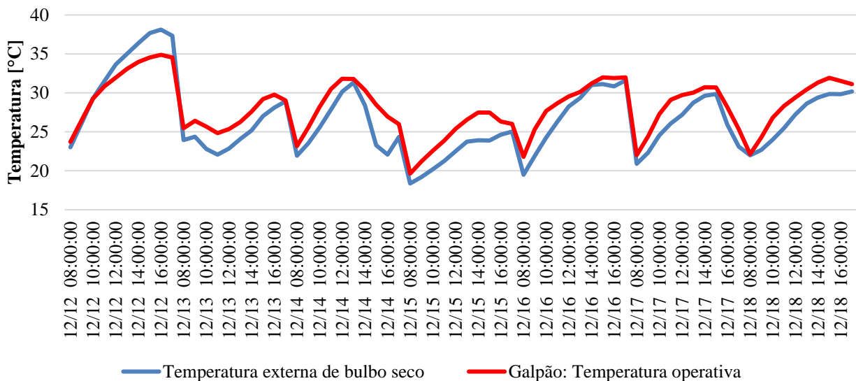
Figura 3. Comportamento da temperatura operativa no Caso 1 para semana típica de verão de projeto.
