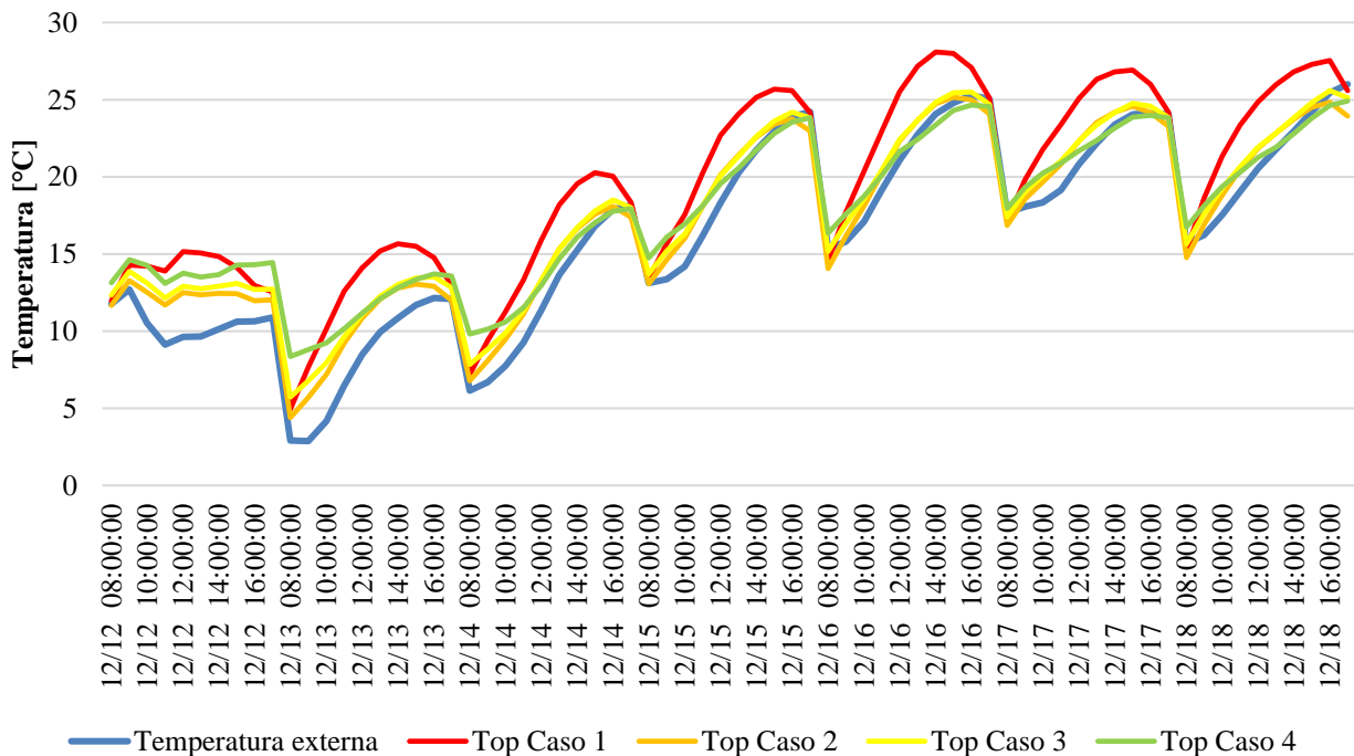
Figura 7. Comparação da temperatura operativa dos casos de envoltória para a semana típica de inverno de projeto.
