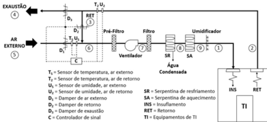
Figura 2. Diagrama de um sistema típico de direct airside free cooling . Adaptado de Lee e Chen (2013).
