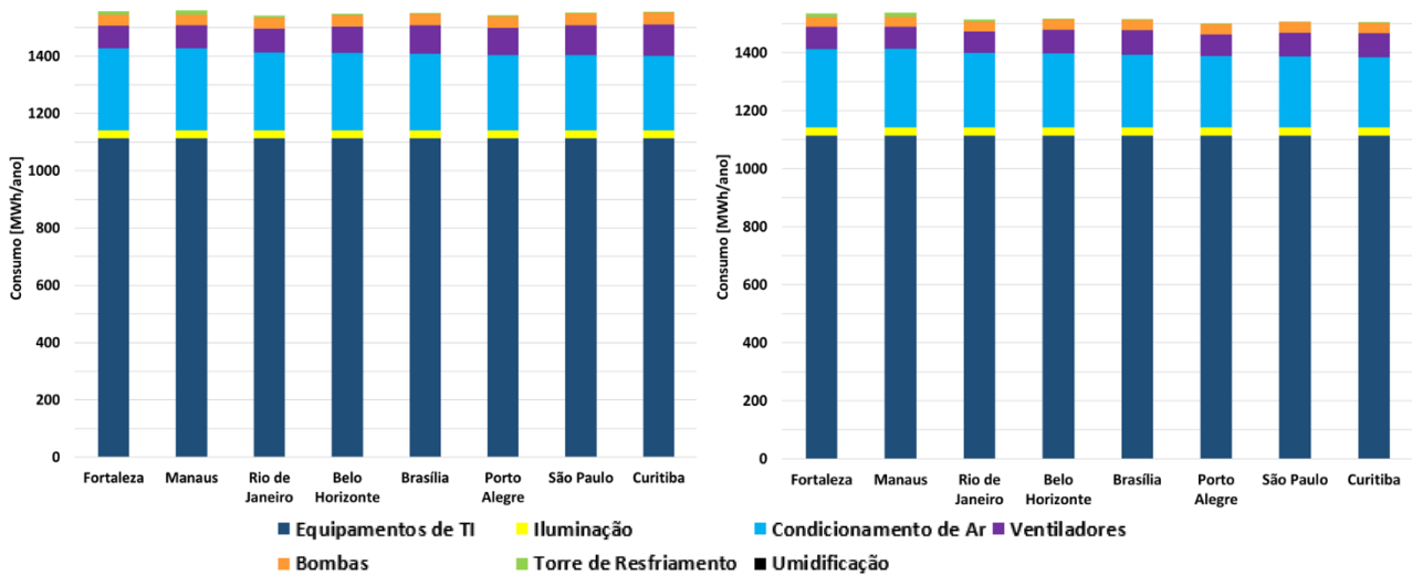
Figura 3. Consumo anual sob a Classe Recomendada e A4, sem aplicação de free cooling .
