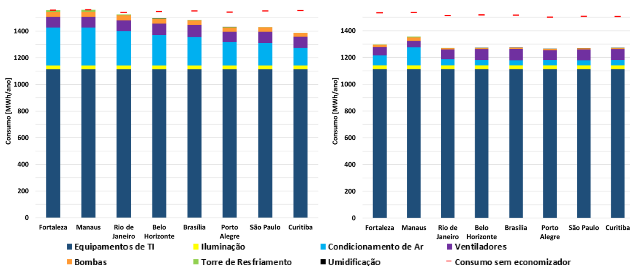
Figura 4. Consumo anual sob a Classe Recomendada e A4, com utilização de free cooling .
