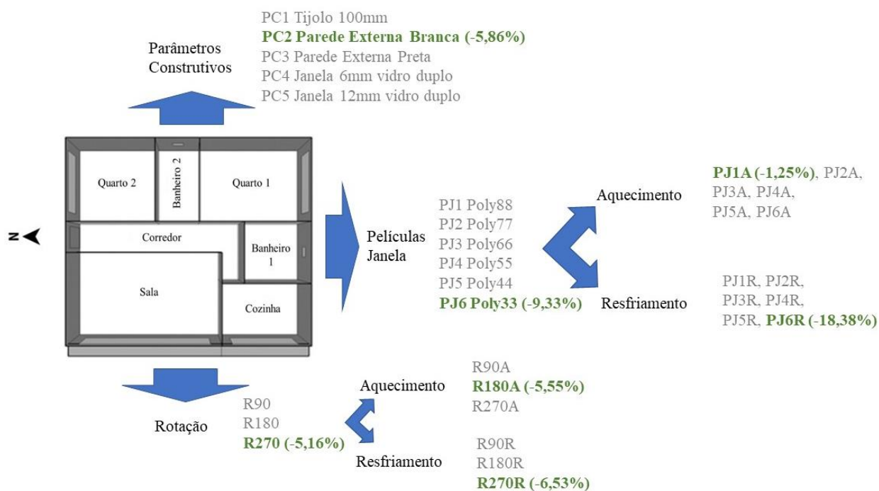
Figura 7. Esquema contendo a casa padrão, os cenários simulados com seus respectivos códigos de identificação, com destaque para aqueles que apresentaram os melhores resultados.
