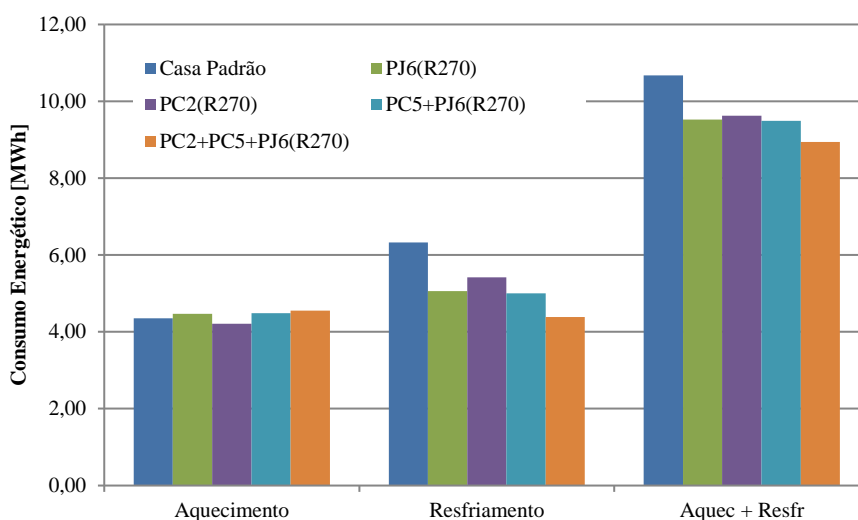
Figura 8 – Consumo energético da edificação para diferentes cenários combinados.
