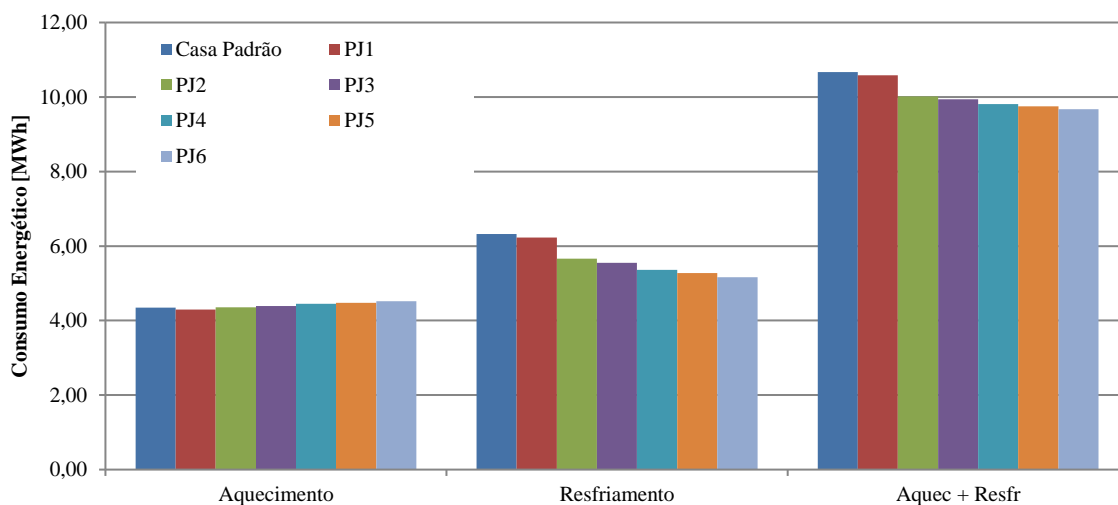
Figura 5 – Consumo energético da edificação para diferentes cenários em função das cargas de aquecimento e resfriamento.
