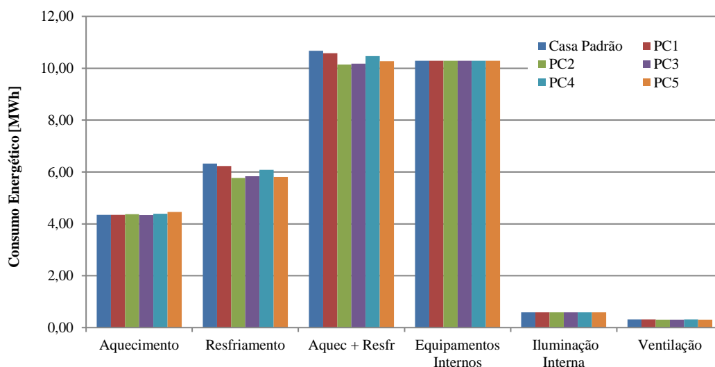
Figura 4 – Consumo energético da edificação para diferentes cenários em função das cargas.
