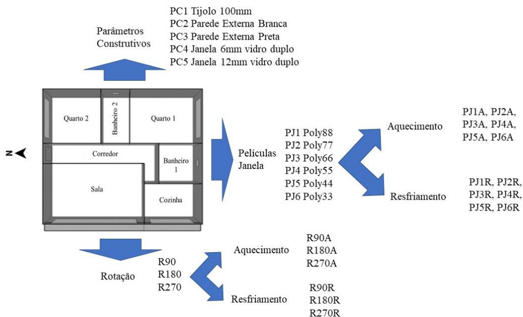
Figura 3. Esquema contendo a casa padrão e os cenários simulados com seus respectivos códigos de identificação.
